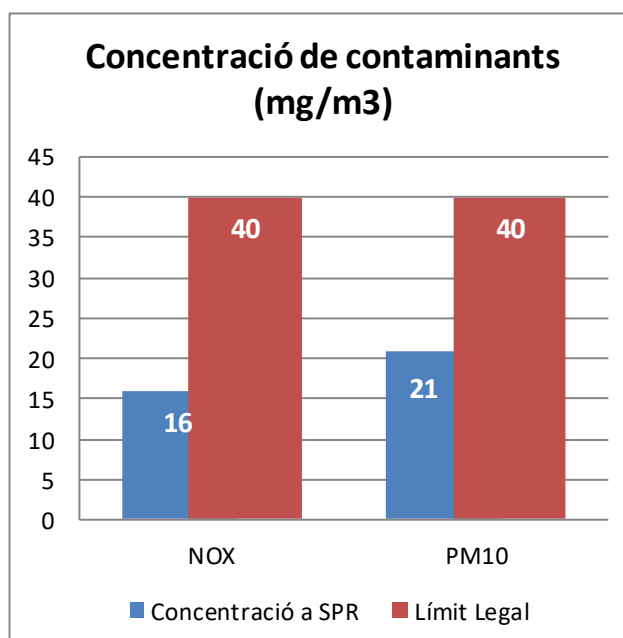
Fig. 79: Immissions de contaminants. Font: AIM, en base a dades de Direcció General de Qualitat Ambiental del DTES.
