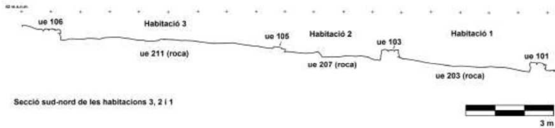
Figura 36. Secció sud-nord de les habitacions 3, 2 i 1
